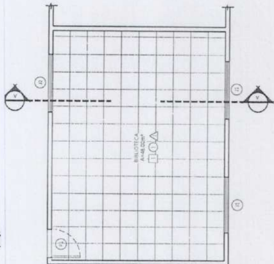
02 PLANTA BAIXA - LAYOUT ESCALA 1/75
