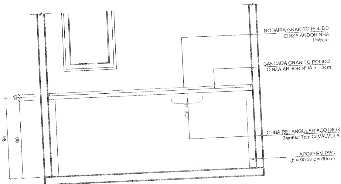
02 ELEVÇÃO ESCALA 1:25
