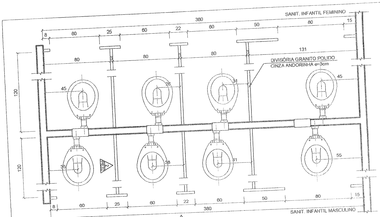
01 PLANTA ESCALA 1:25
