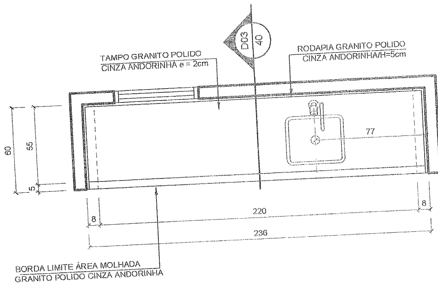
01 PLANTA ESCALA 1:25
