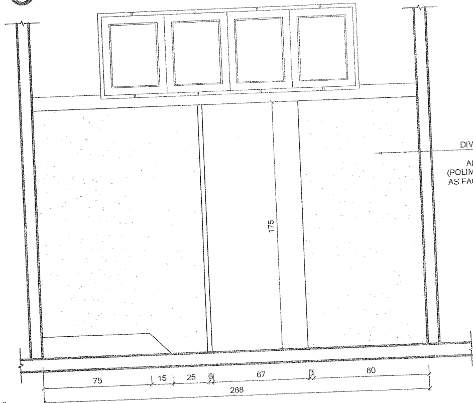
02 CORTE AA ESCALA 1:25
