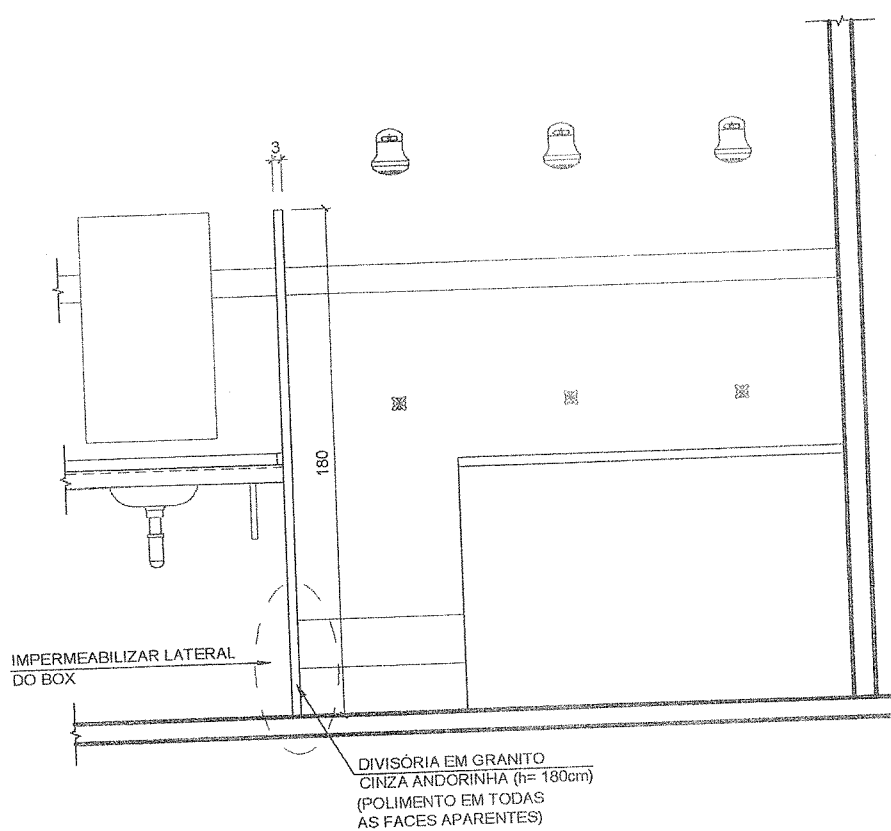
02 ELEVAÇÃO 1 ESCALA 1:25
