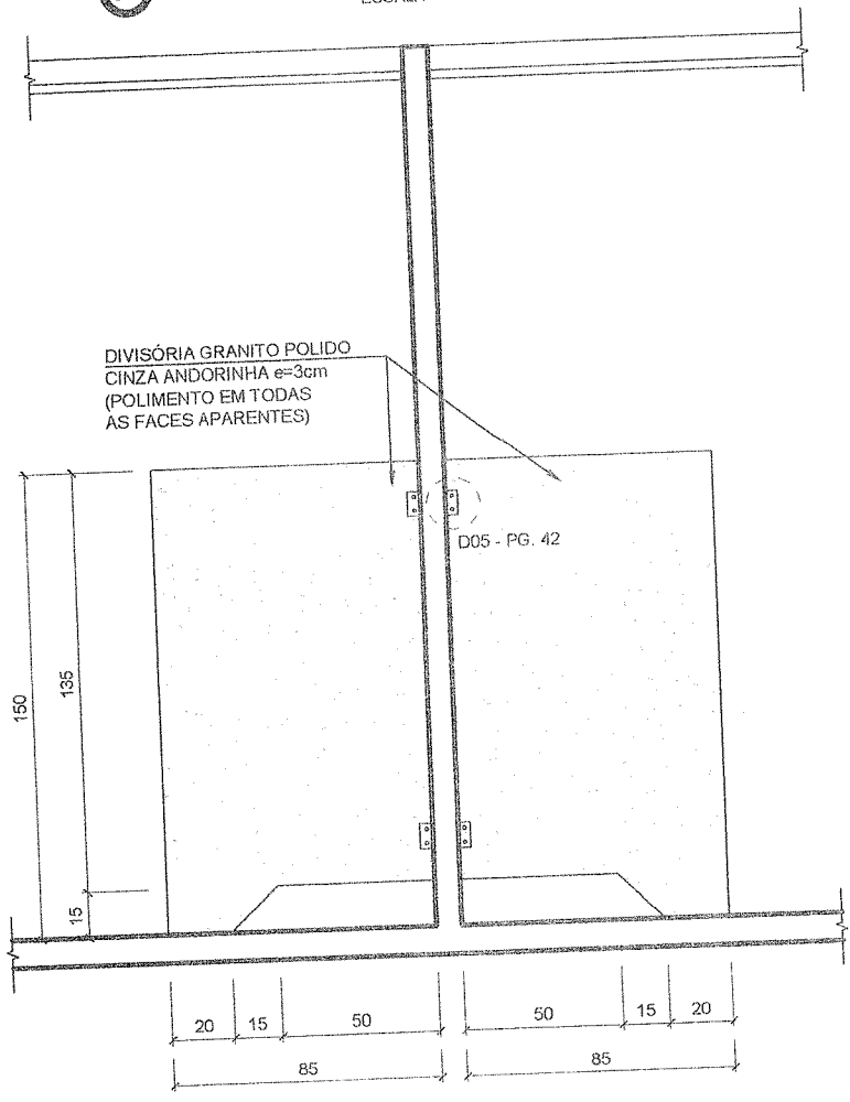
ELEVACÃO ESCALA 1:25
