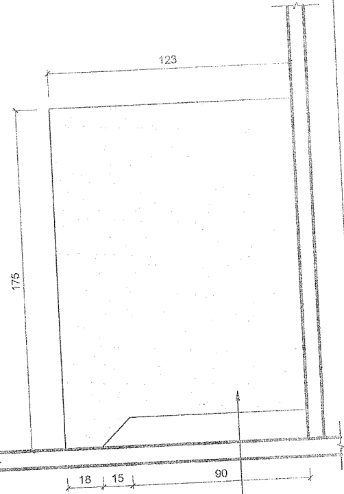
03 ELEVACÃO 2 ESCALA 1:25
