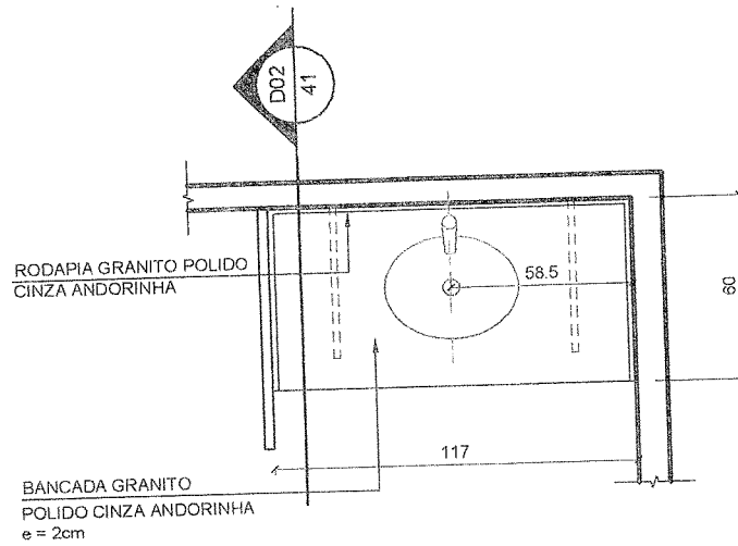
01 PLANTA ESCALA 1:25
