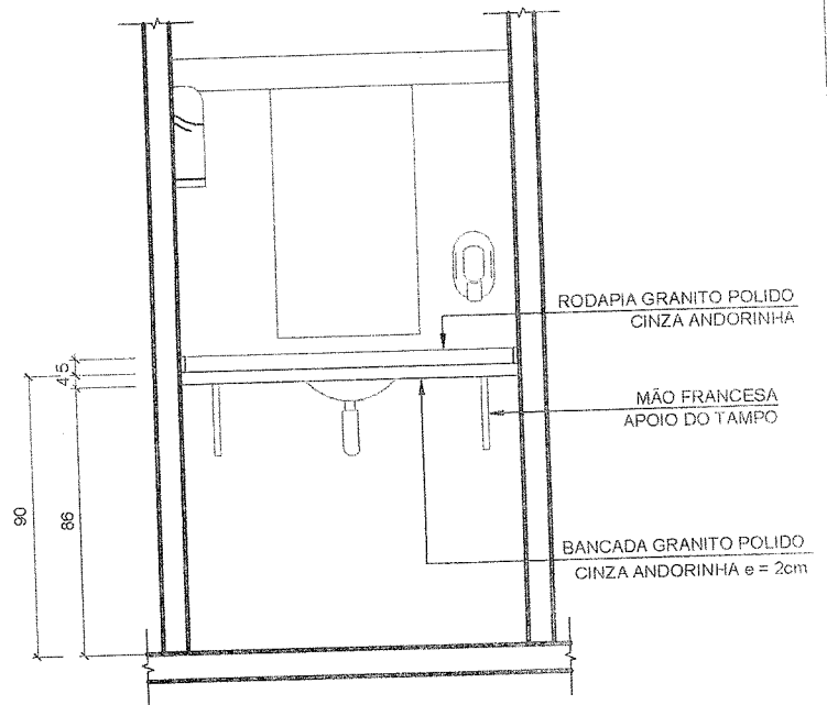
04 B10 - ELEVÇÃO ESCALA 1:25
