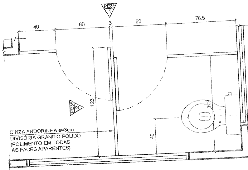
01 PLANTA ESCALA 1:25
