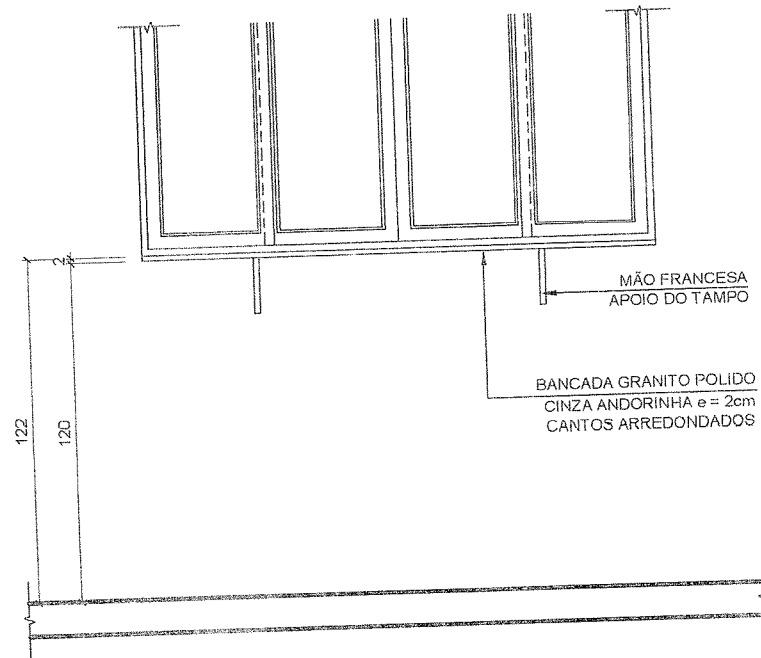
02 ELEVAÇÃO ESCALA 1:25
