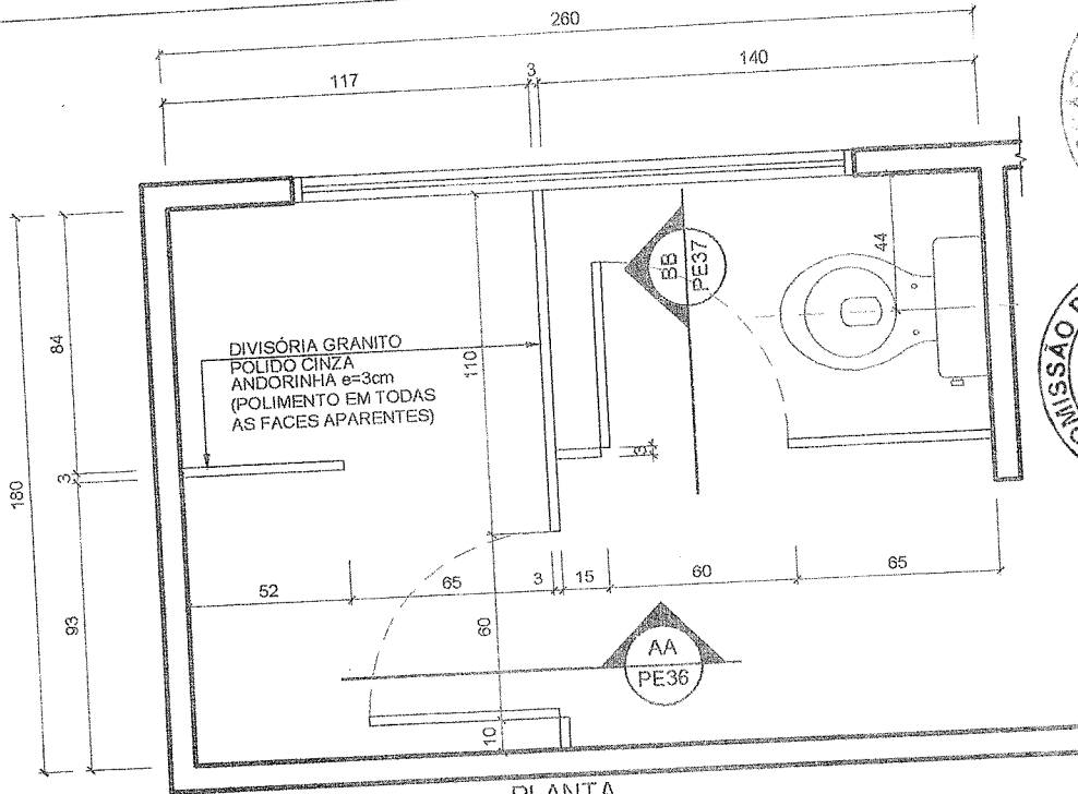
01 PLANTA ESCALA 1:25
