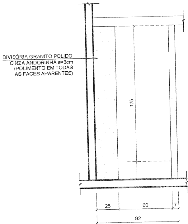
02 CORTE CC ESCALA 1:25
