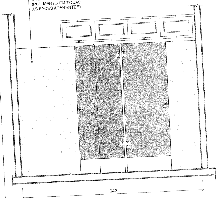
02 ELEVACÃO 1 ESCALA 1:25
