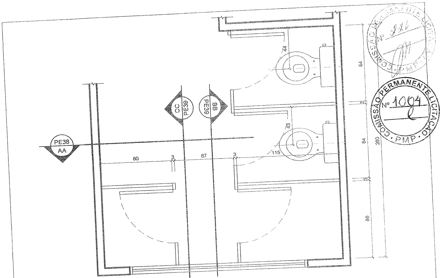
01 PLANTA ESCALA 1:25
