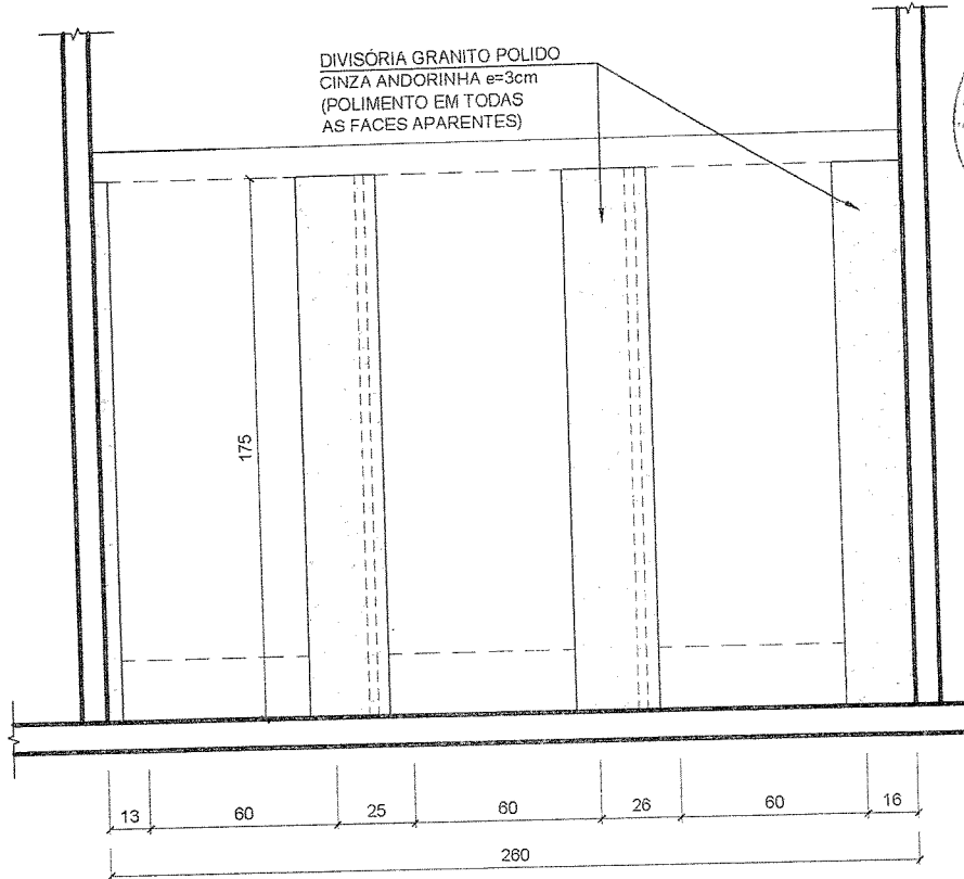
01 CORTE BB ESCALA 1:25
