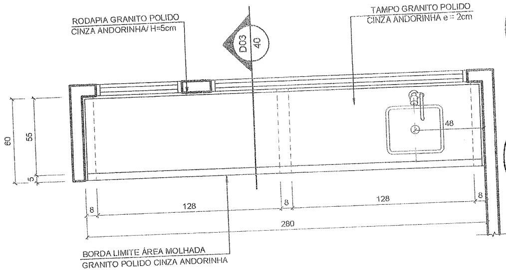
01 PLANTA ESCALA 1:25
