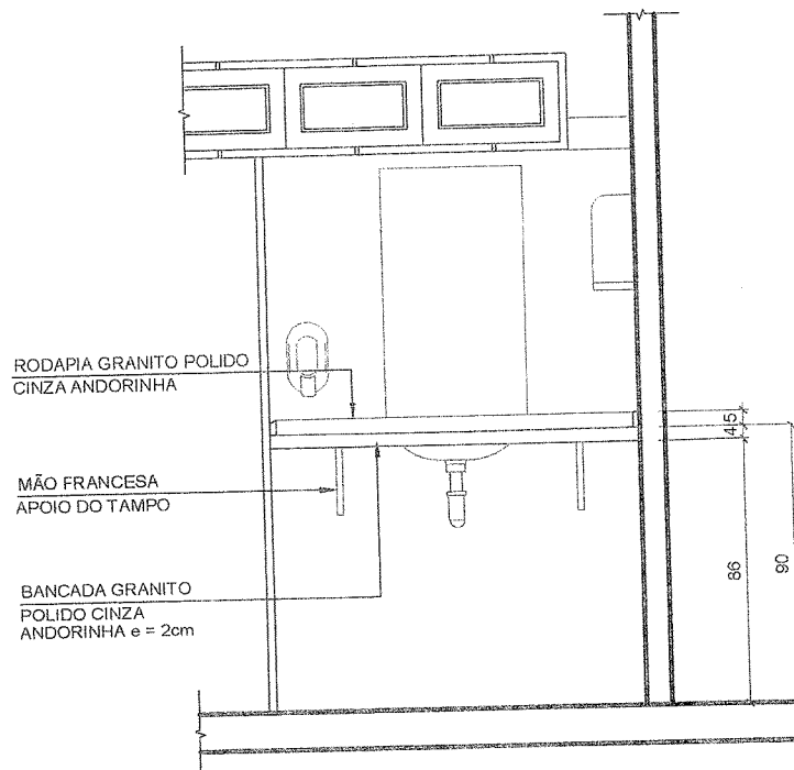
02 ELEVÇÃO ESCALA 1:25
