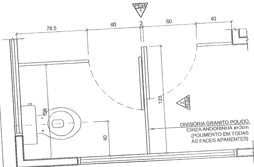
01 PLANTA ESCALA 1:25
