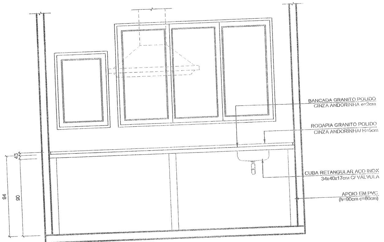
02 ELEVACÃO ESCALA 1:25
