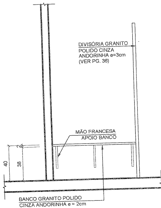
03 B21 - ELEVÇÃO ESCALA 1:25
