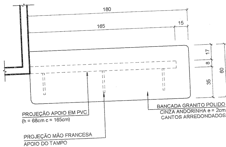
01 PLANTA ESCALA 1:25
