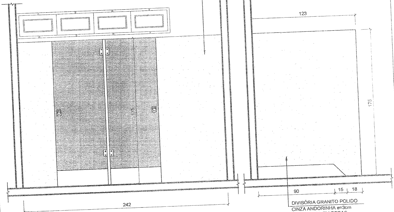
03 ELEVAÇÃO 2 ESCALA 1:25
