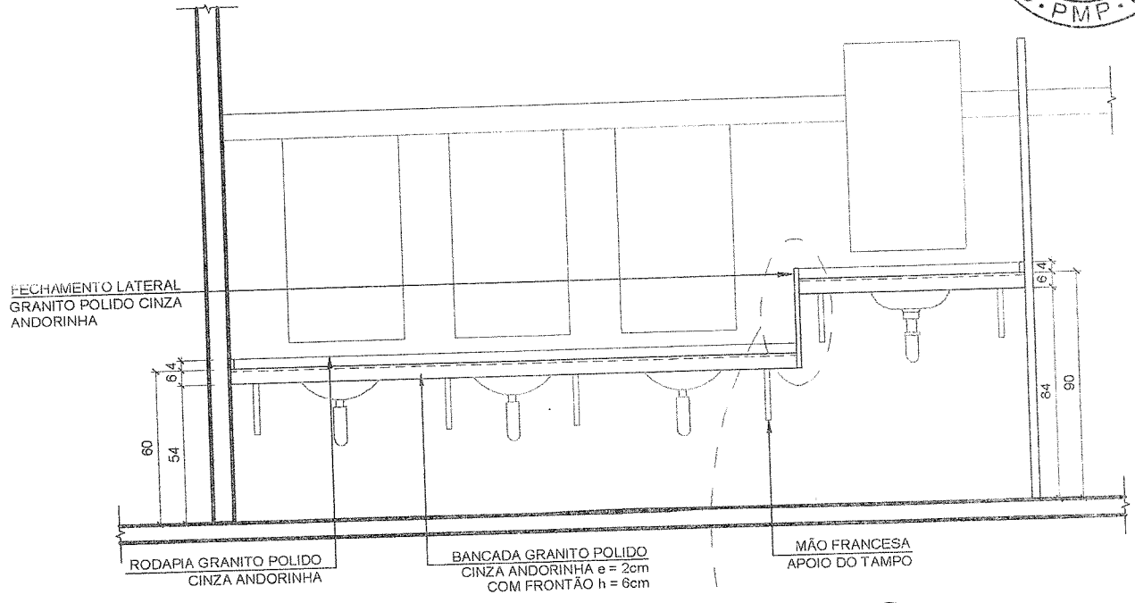
02 ELEVAÇÃO ESCALA 1:25
