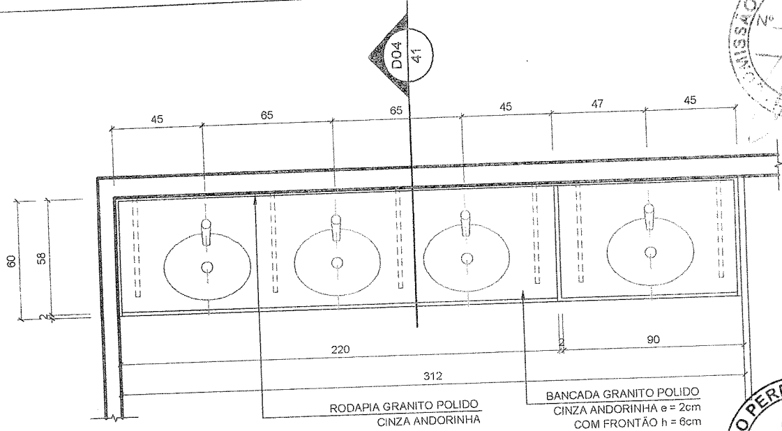
01 PLANTA ESCALA 1:25
