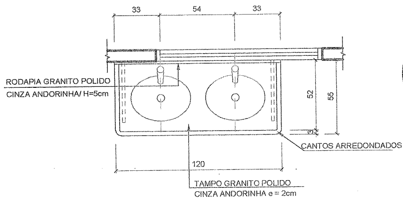
01 PLANTA ESCALA 1:25
