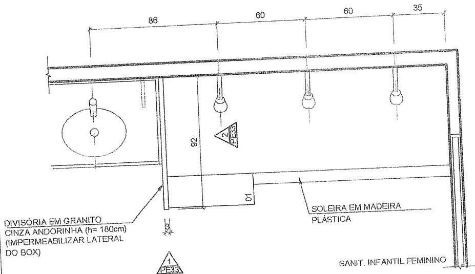
01 PLANTA ESCALA 1:25
