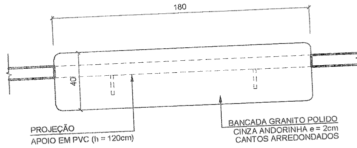
01 PLANTA ESCALA 1:25
