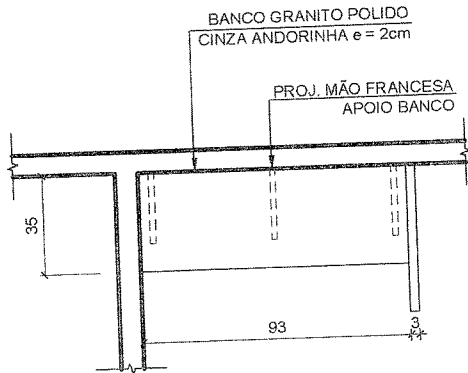
01 B21 - PLANTA ESCALA 1:25
