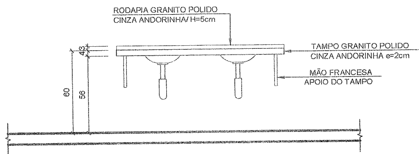
02 ELEVAÇÃO ESCALA 1:25
