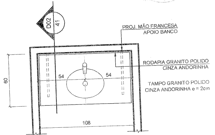
02 B10 - PLANTA ESCALA 1:25
