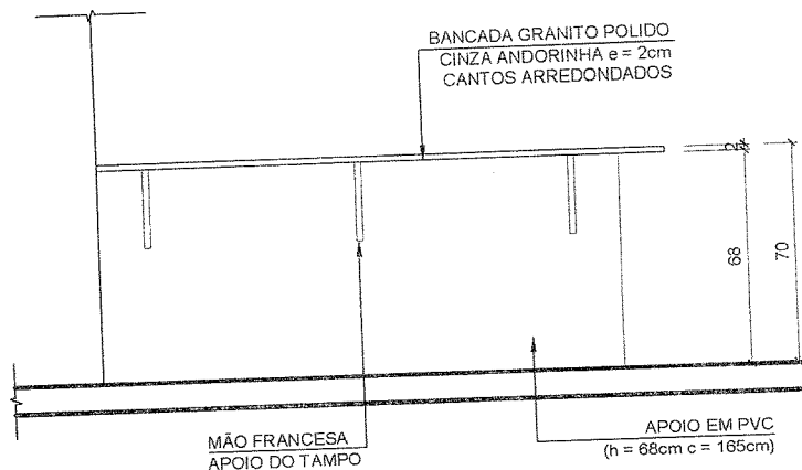
02 ELEVACÃO ESCALA 1:25
