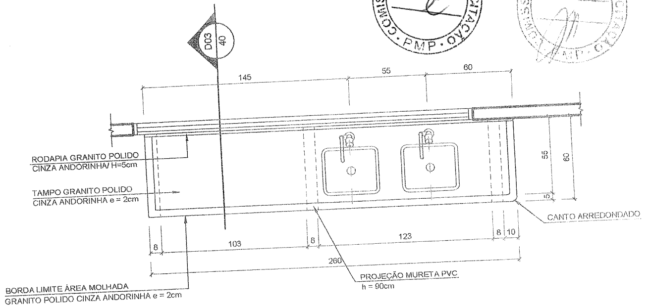
01 PLANTA ESCALA 1:25
