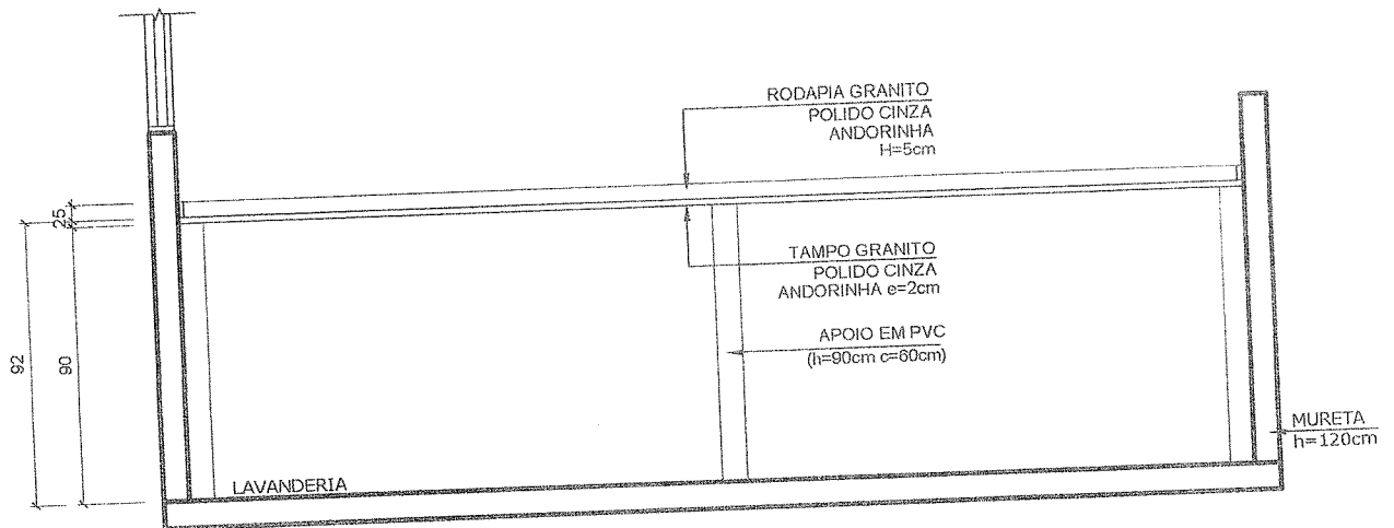
02 ELEVACÃO ESCALA 1:25
