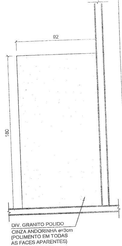
03 ELEVAÇÃO 2 ESCALA 1:25
