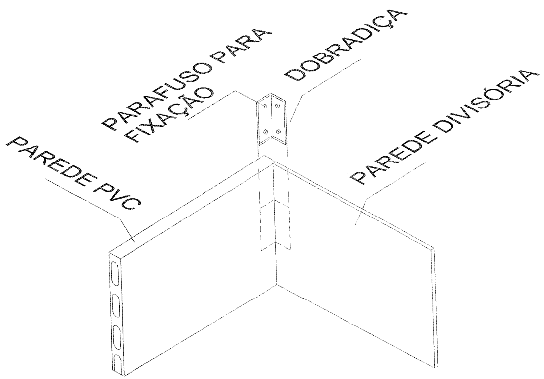
01 D05 - DIVISÓRIAS DETALHE FIXAÇÃO ESCALA —
