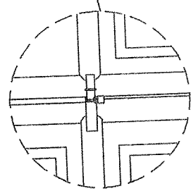
DETALHE TRAVA COM PORTA CADEADO ESCALA 1:10 02
