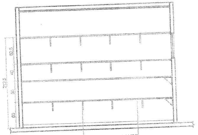
MÃO FRANCESA METÁLICA PINTURA COR CINZA PRATELEIRA EM MDF BRANCO 25mm
