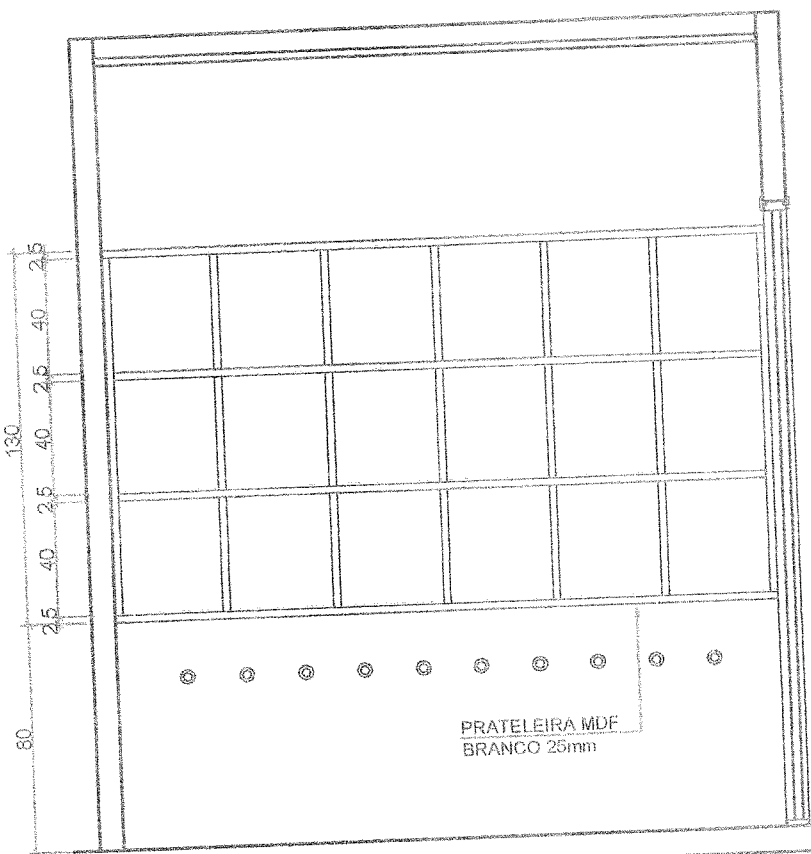
02 ELEVAÇÃO ESCALA 1:25
