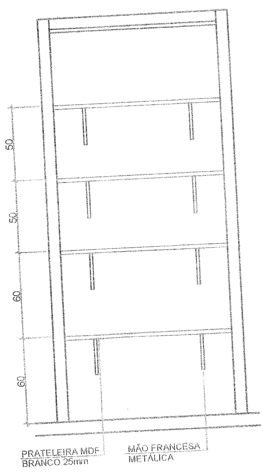
02 ELEVÇÃO ESCALA 1:25
