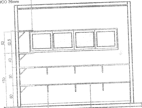
MÃO FRANCESA METÁLICA PINTURA COR CINZA PRATELEIRA EM MDF BRANCO 25mm CANTONEIRA METÁLICA PINTURA COR CINZA
