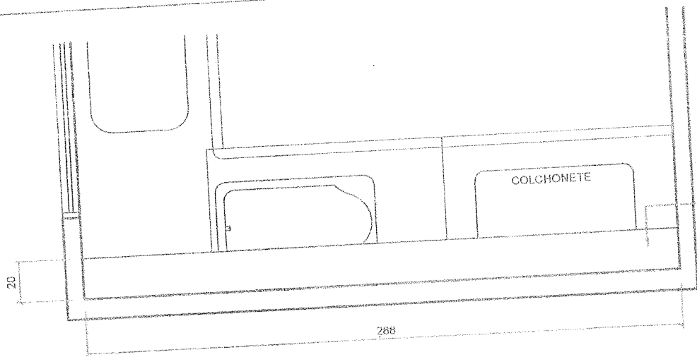
01 PLANTA ESCALA 1:25
