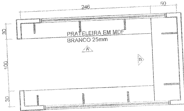
01 PLANTA ESCALA 1:40
