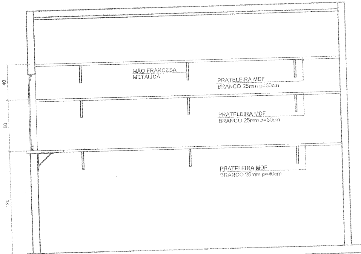
02 ELEVACÃO ESCALA 1:25
