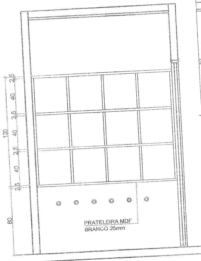
02 ELEVÇÃO ESCALA 1:25
