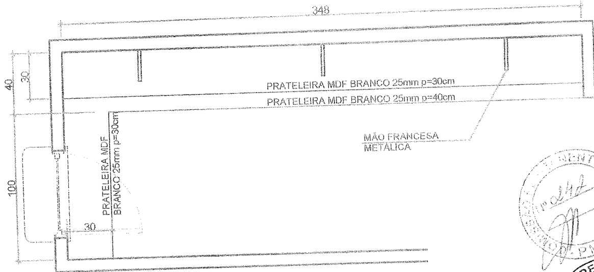
01 PLANTA ESCALA 1:25
