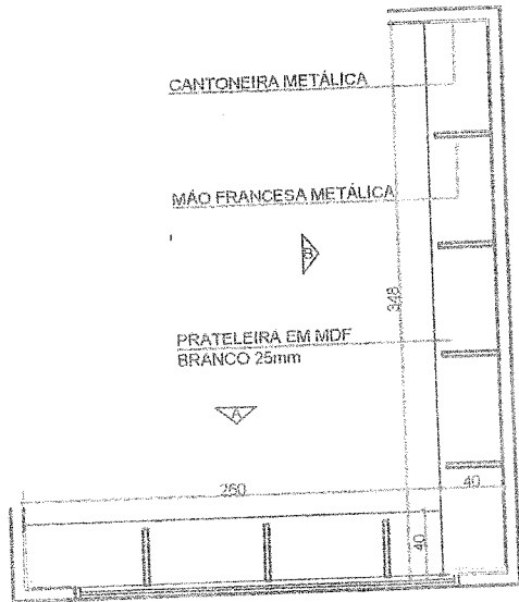
01 PLANTA ESCALA 1:50
