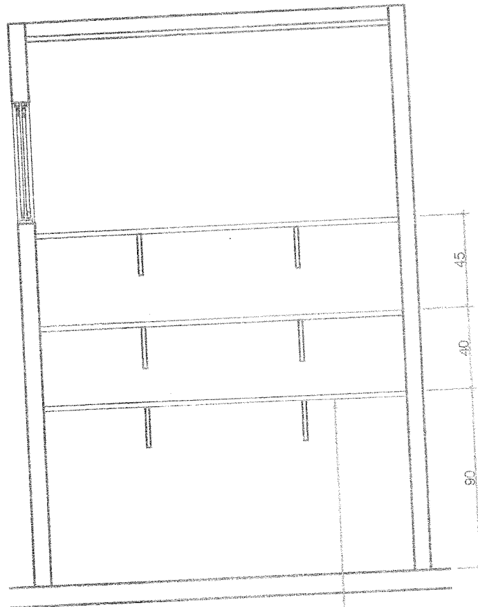
01 PLANTA ESCALA 1:25
