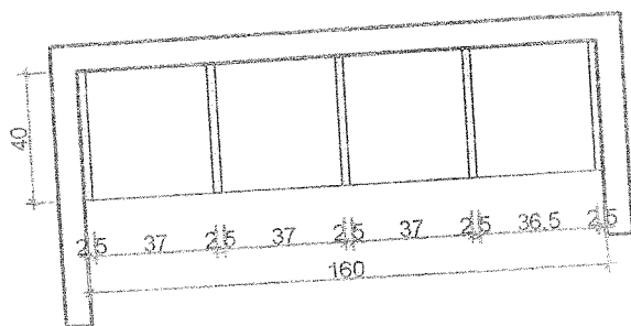
01 PLANTA ESCALA 1:25
