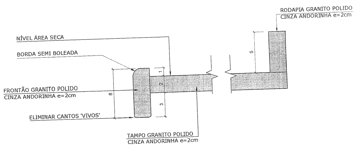
02 D04 - BANCADAS DETALHE FRONTÃO ESCALA 1:2,5
