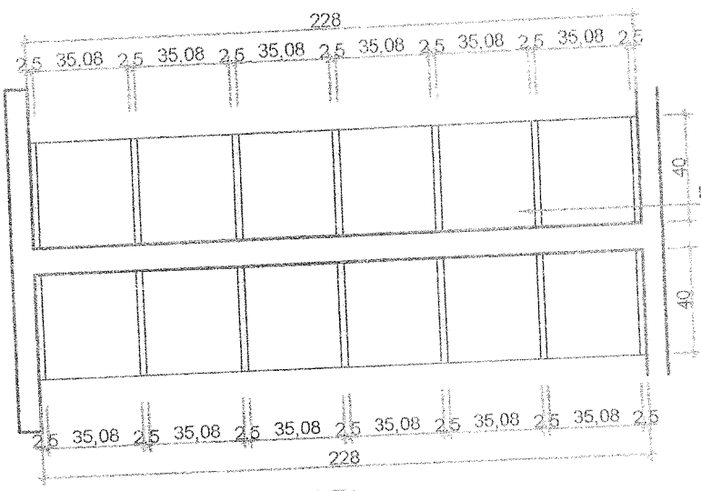
01 PLANTA ESCALA 1:25
