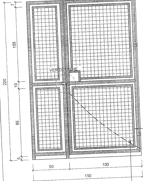
ELEVAÇÕES ESCALA 1:25
